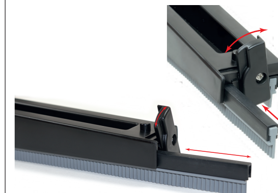
Changement facile et sans outil de la lèvre. N° article 102.126
