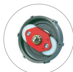
Réducteur à satellites et planétaire (L16)
